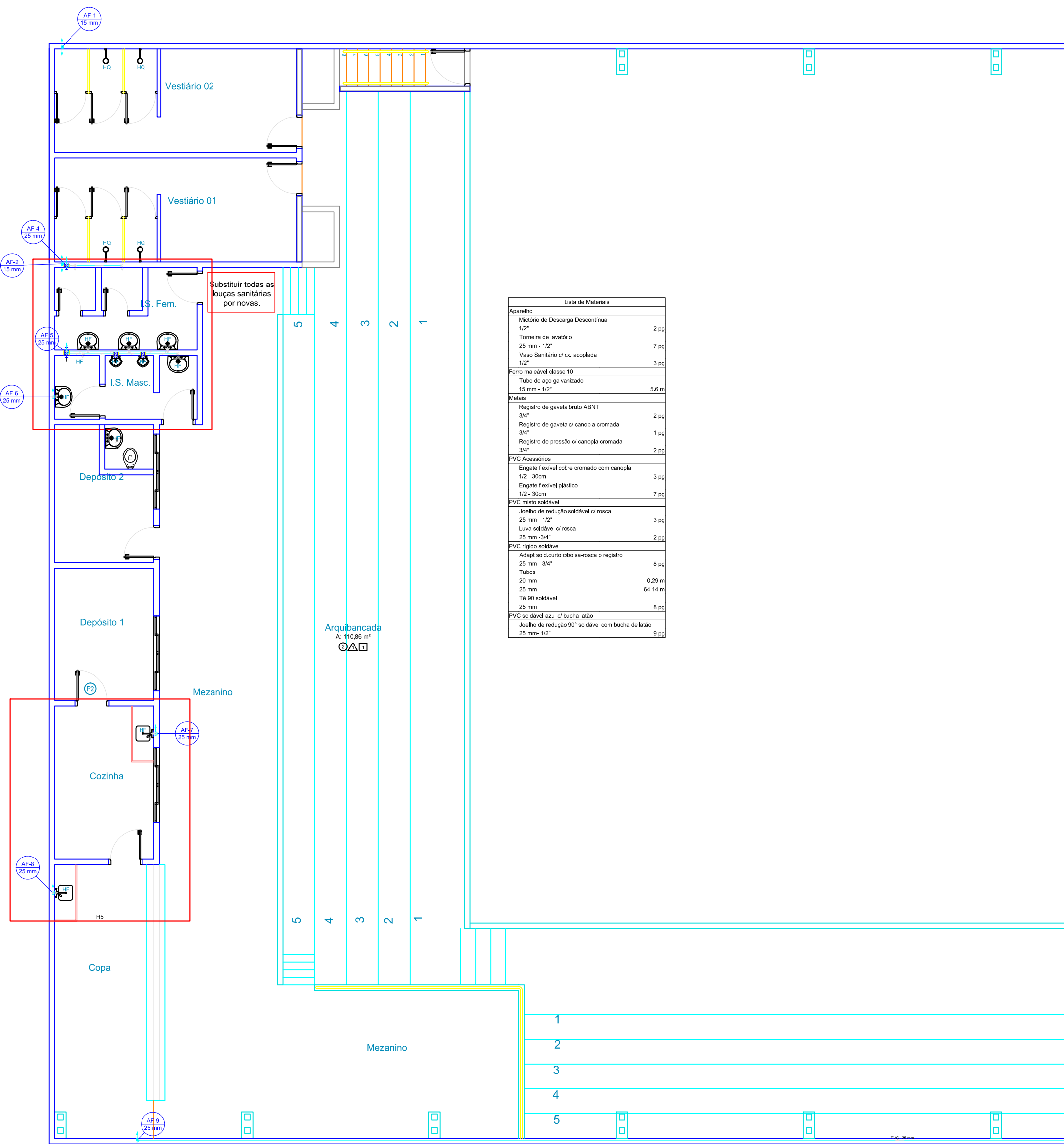
BANHEIROS - HIDRÁULICO - PLANTA BAIXA Escala 1:100
